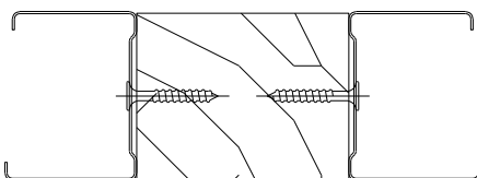
2- Montant bois 58x46mm pris en sandwich entre deux montants M48 dos à dos
