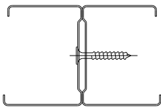
1- Deux montants M48 dos à dos
