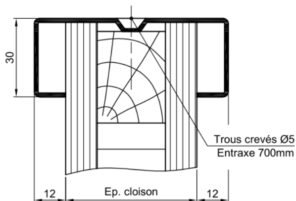
CLOISON ALVEOLAIRE
