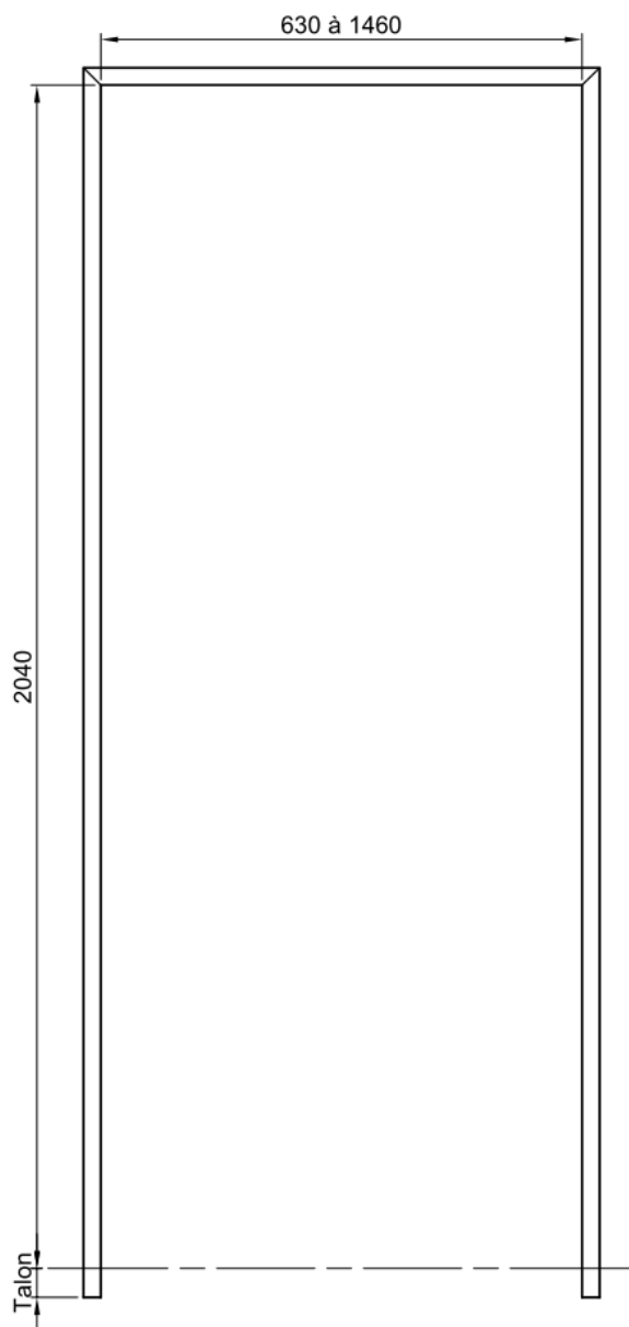
CLOISON ALVEOLAIRE
