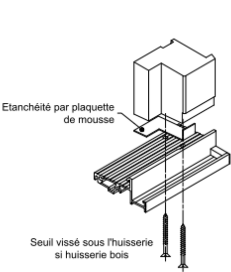
Sur Huisserie Bois
