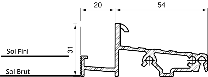
Sur Huisserie Bois
