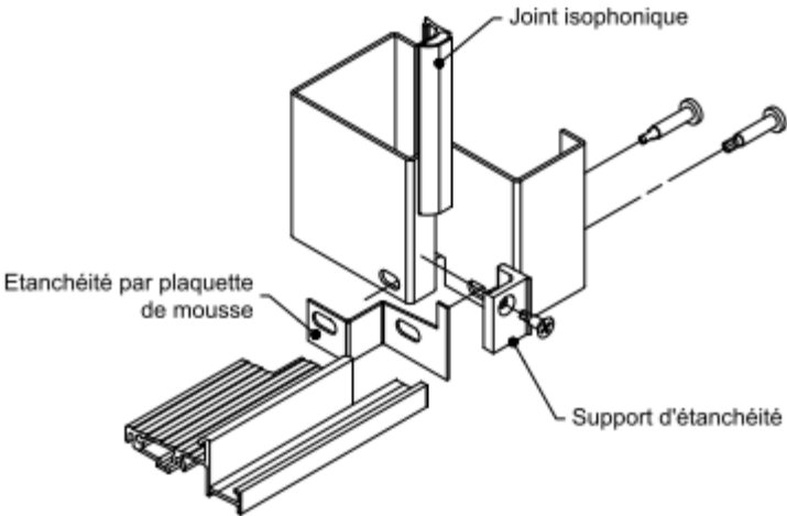
FIXATION HUISSERIE MÉTALLIQUE ISOPHONIQUE
