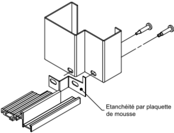
Sur Huisserie Métallique
