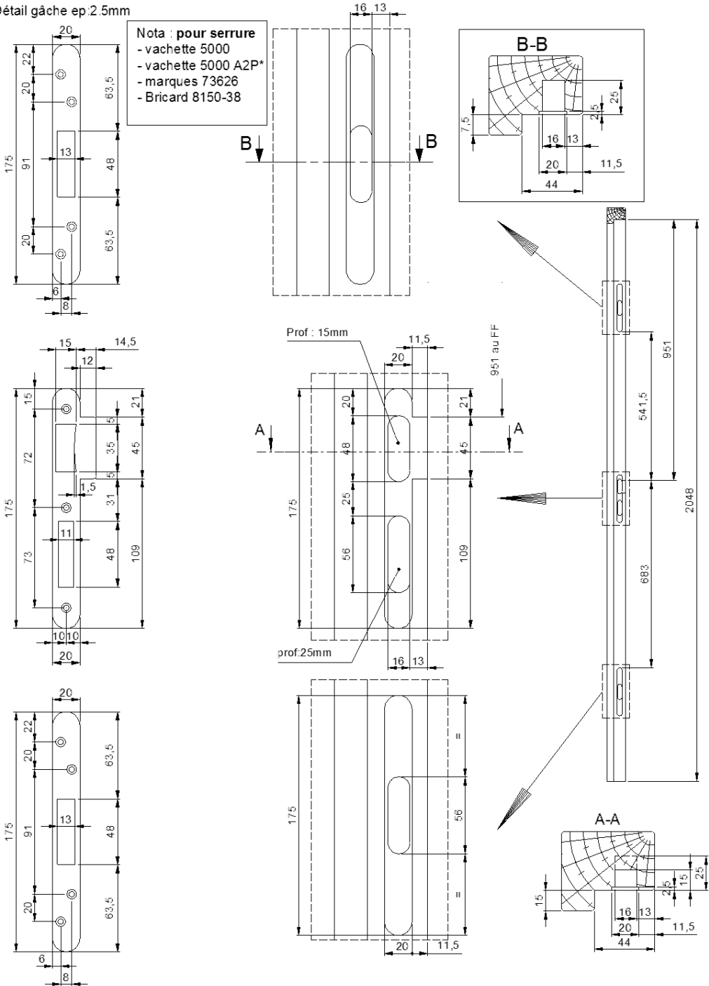
Détail gâche ep 2.5mm
