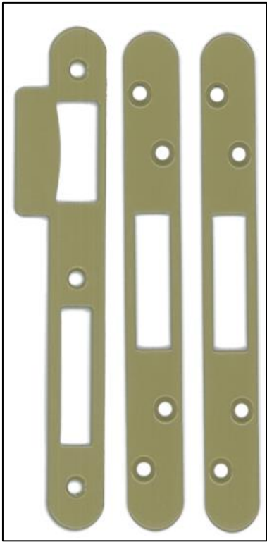
Détail gâche ep 2.5mm
