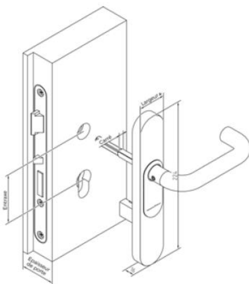
Modèle pour Montage SNAP IN
