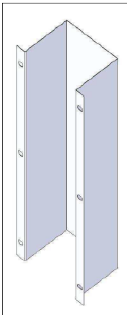
Carter de protection Largeur : 330mm (250+40+40) Epaisseur : 206mm
