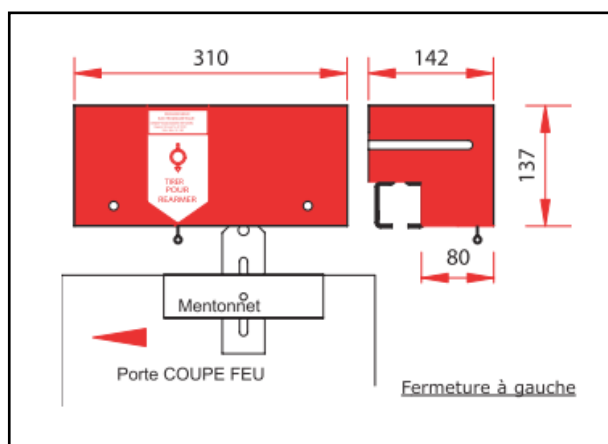
Déclencheur électromagnétique
