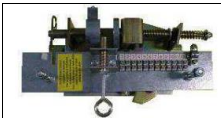
Déclencheur électromagnétique
