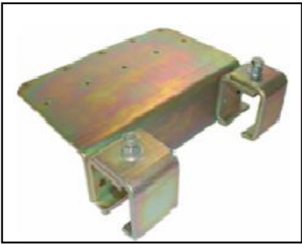
Support d'amortisseur
