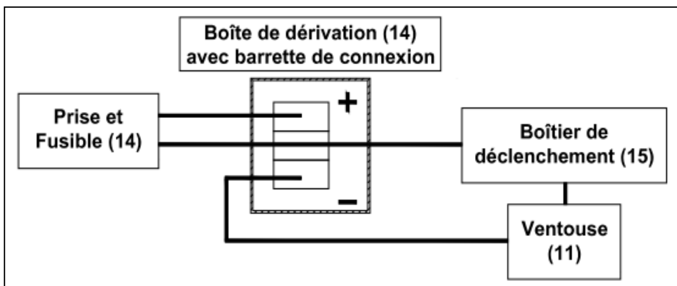
Principe du branchement électrique
