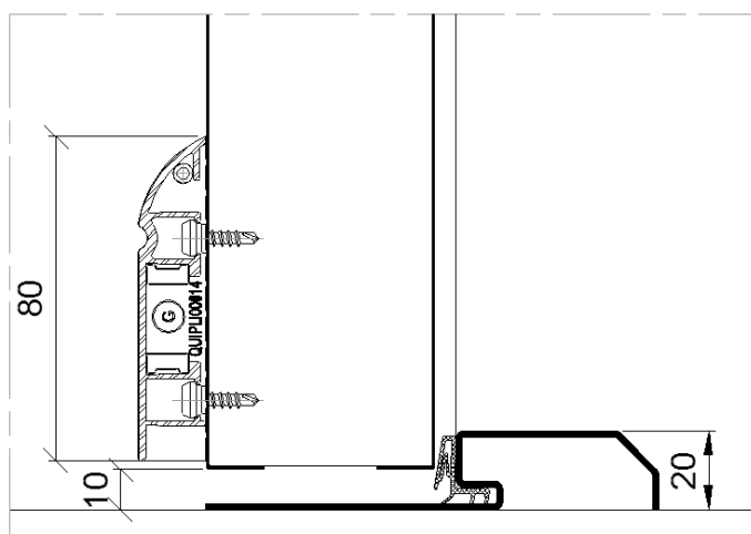
Pose de la plinthe rejet d'eau côté paumelles avec seuil suisse
