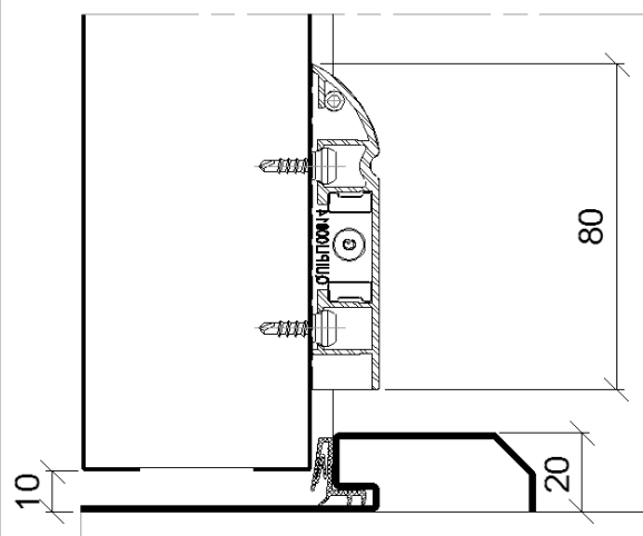
Pose de la plinthe rejet d'eau côté opposé paumelles avec seuil suisse
