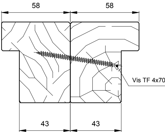
Assemblage dos à dos
