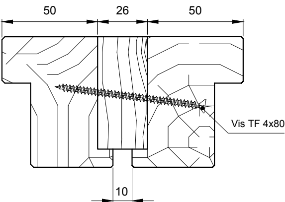
Poteau de fin de cloison
