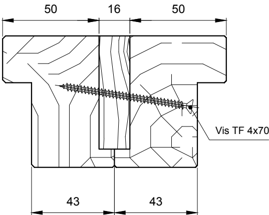
Assemblage avec fourrure de liaison
