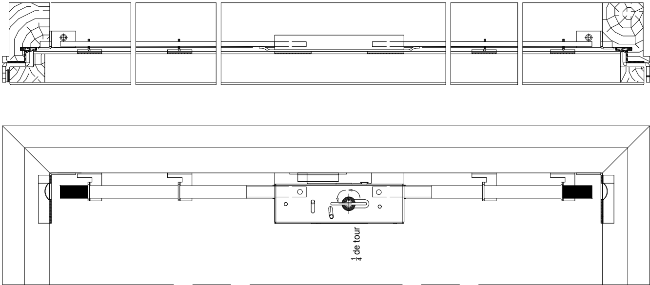
Bloc-gaine ouvert
