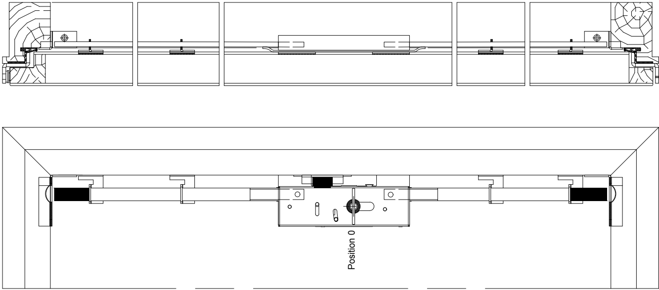
Bloc-gaine fermé mais non verrouillé
