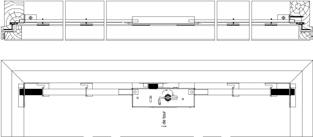
Bloc-gaine verrouillé
