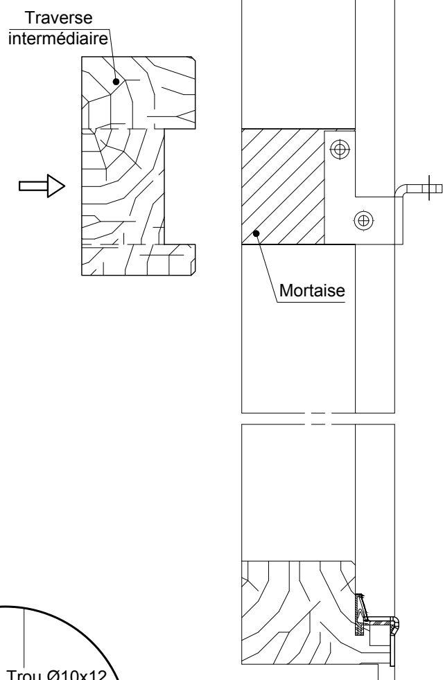
Etape 2 Mise en place de la traverse intermédiaire
