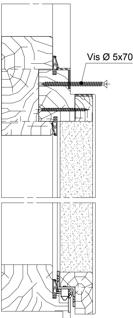
Etape 4 Fixation de l'allège sur la traverse intermédiaire
