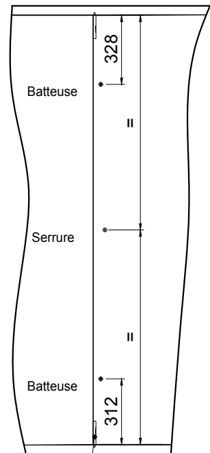
BLOCS-GAINES GAZ 2 batteuses + serrure BCS
