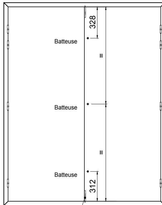
BLOCS-GAINES ELECTRIQUE, EAU, TéléCOM, SG, etc. 3 batteuses
