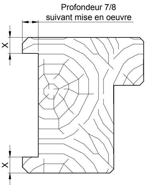
Rainure à brique
