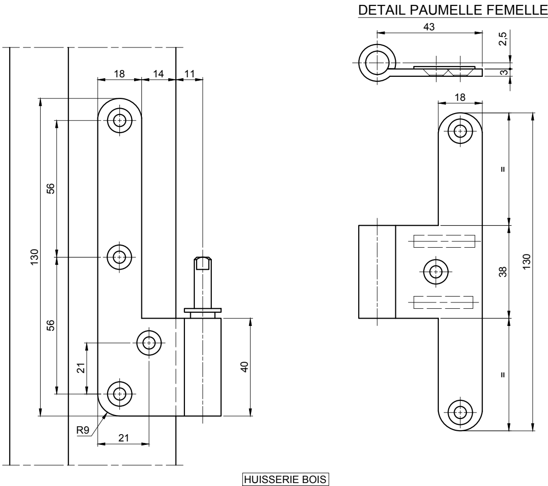
HUISSERIE BOIS
