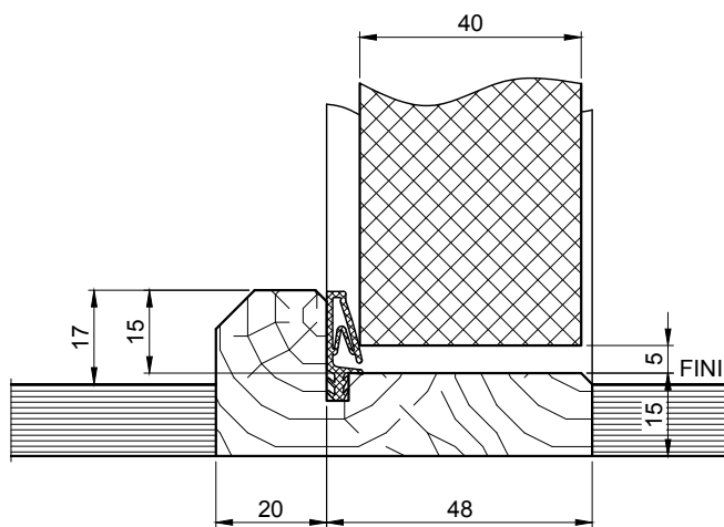
SEUIL SUISSE ISO BOIS
