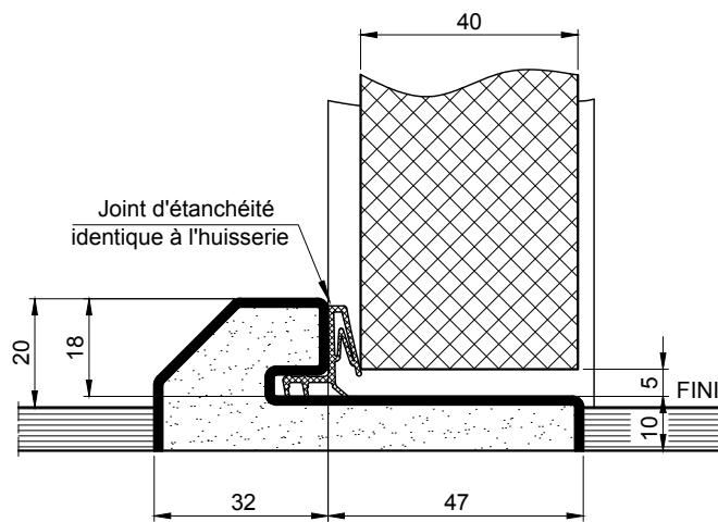
SEUIL SUISSE ISO ACIER
