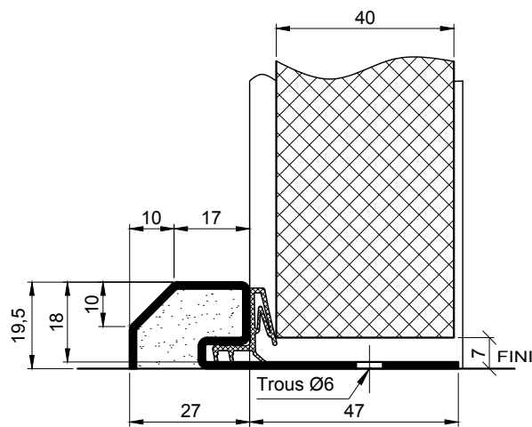
SEUIL SUISSE ISO ACIER RAPPORTE REHABILITATION SANS RETOUR
