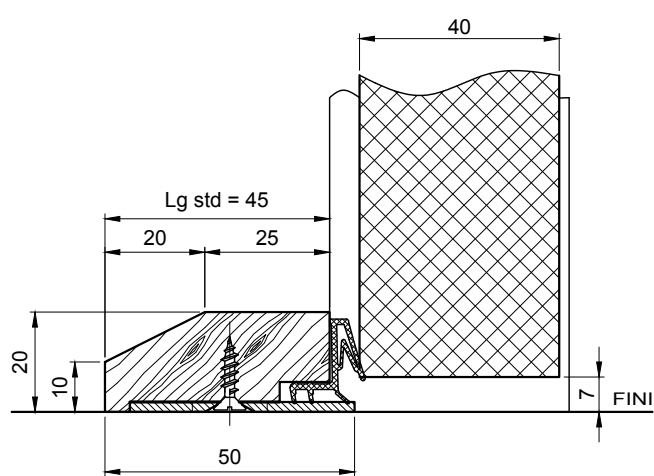
SEUIL SUISSE ISO BOIS RAPPORTE REHABILITATION SANS RETOUR
