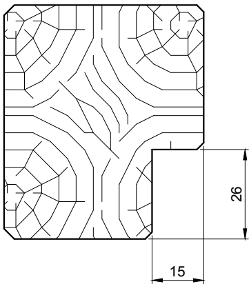
Feuillure Type A
