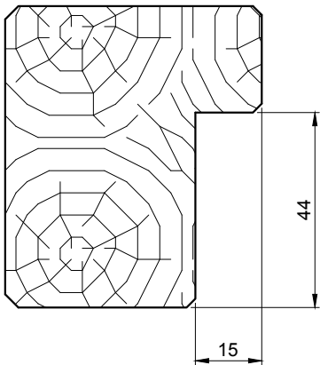
Feuillure Type C
