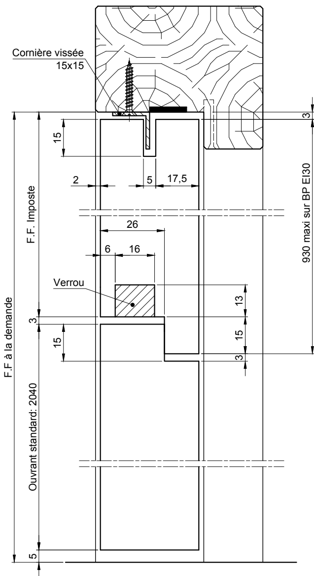
FIXATION PAR VERROU
