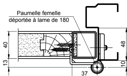
COUPE SUR PAUMELLE DU BAS
