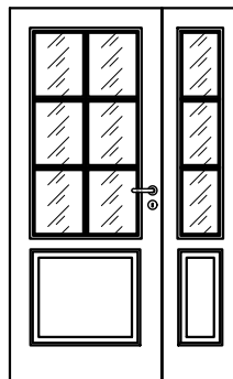
FRANCE TIERCE VITRE AVEC PETITS BOIS
