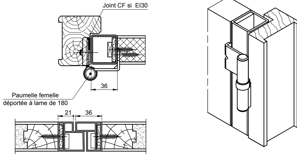
COUPE SUR PAUMELLE DU BAS
