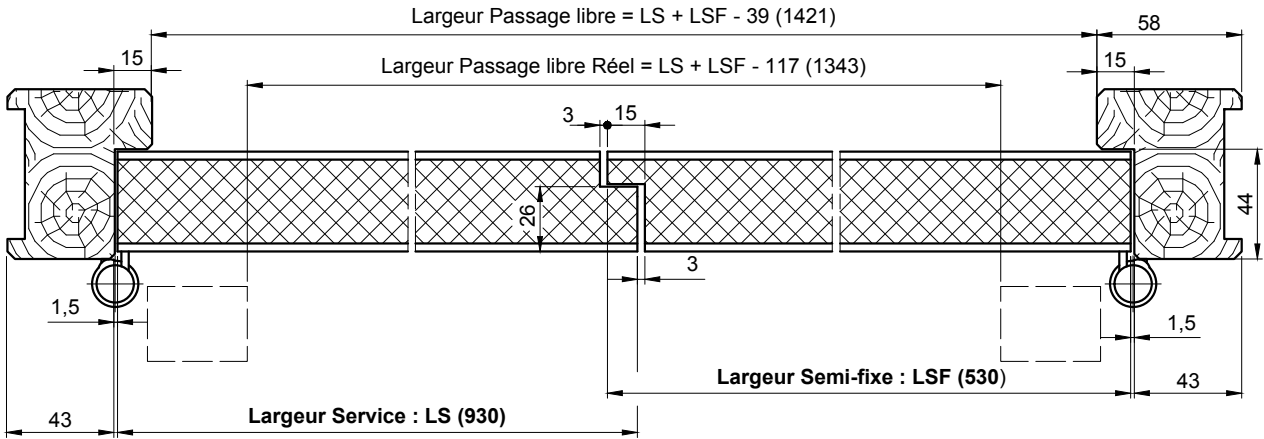
COUPE B-B SUR JOINT ANTI PINCE DOIGTS
