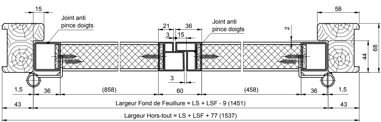
COUPE B-B SUR JOINT ANTI PINCE DOIGTS
