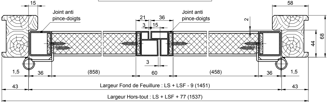
COUPE B-B SUR JOINT ANTI PINCE DOIGTS
