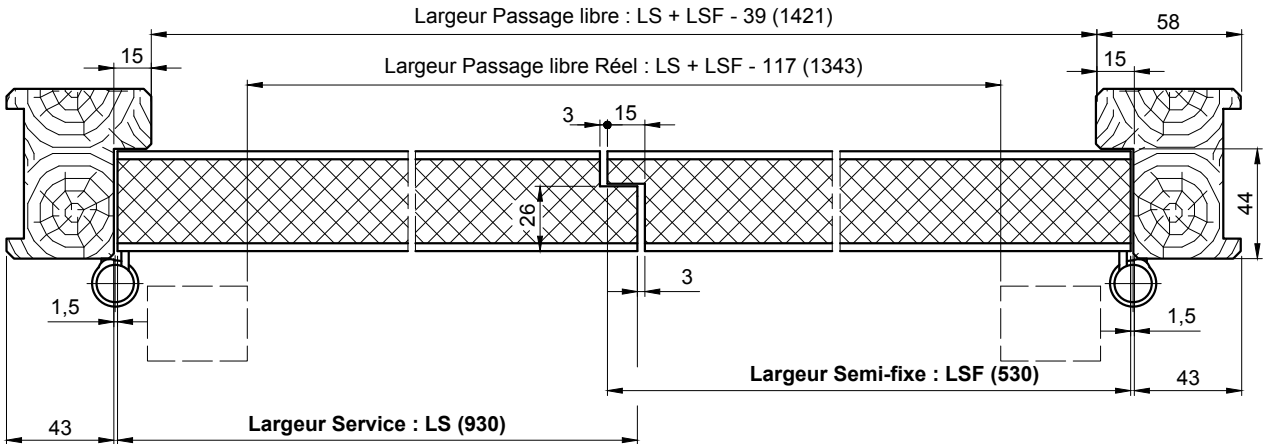
COUPE A-A SUR PARTIE HAUTE
