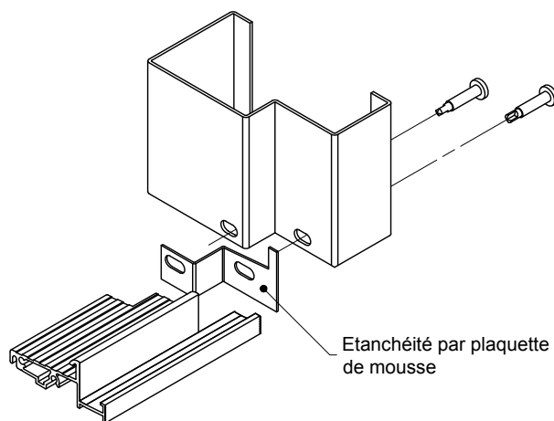
FIXATION HUISSERIE MÉTALLIQUE
