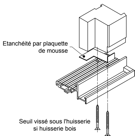
FIXATION HUISSERIE BOIS
