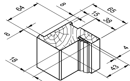
HUISSERIE ISOPHONIQUE SECTION 64x65
