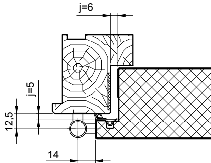
HUISSERIE STANDARD
