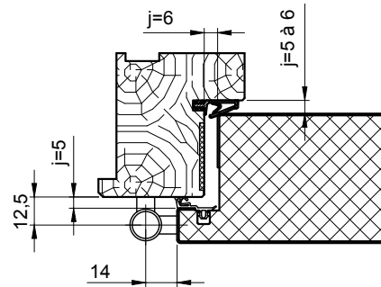
HUISSERIE ISOPONIQUE
