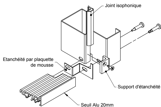
FIXATION HUISSERIE MÉTALLIQUE ISOPHONIQUE
