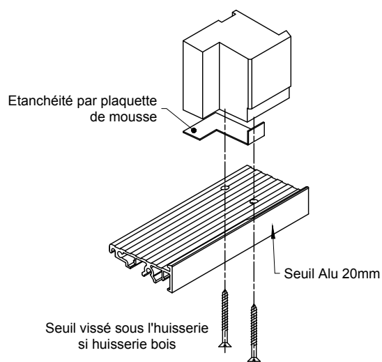
FIXATION HUISSERIE BOIS
