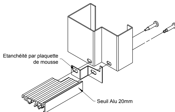
FIXATION HUISSERIE MÉTALLIQUE
