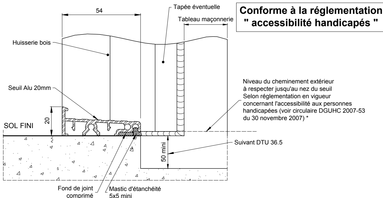
FIXATION HUISSERIE BOIS
