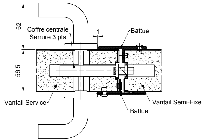
Coupe sur serrure 3 points sur porte 2 vantaux
