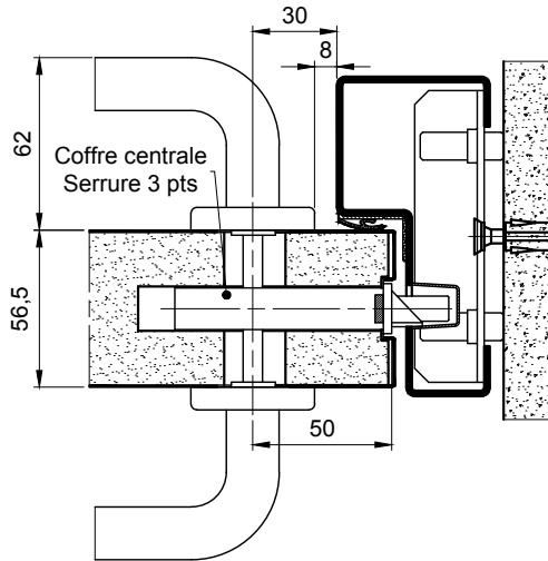
Coupe sur serrure 3 points sur porte 1 vantail
