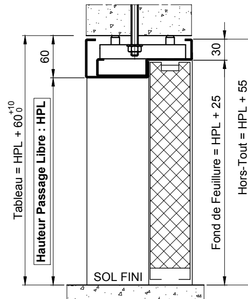
RESERVATION MACONNERIE AVEC BATI A VISSER MONTAGE EN TUNNEL
