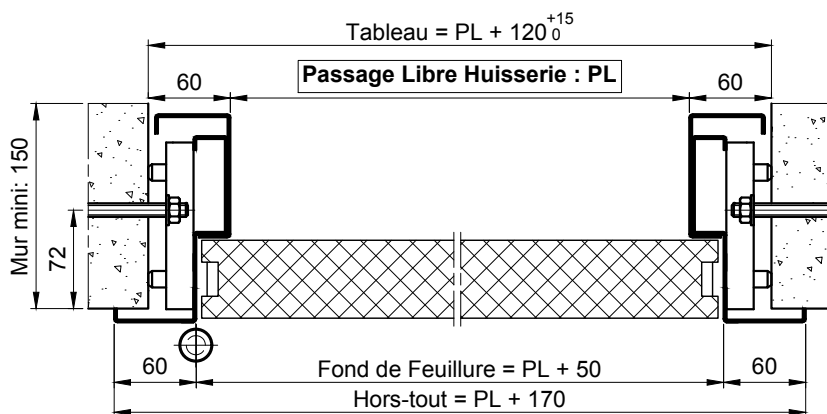
RESERVATION MACONNERIE AVEC BATI A VISSER MONTAGE EN ANGLE (non validé en E120)
