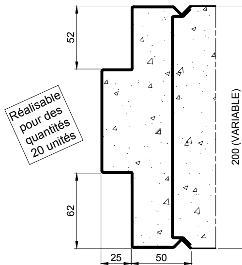
HUISSERIE BANCHEE (TOLE 15/10)
