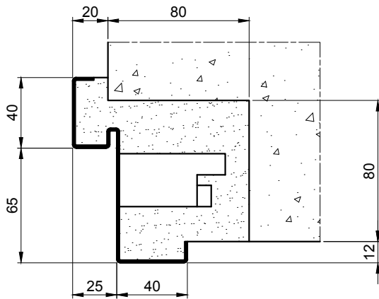
BATI ISOPHONIQUE STANDARD (OUV. INT.)
