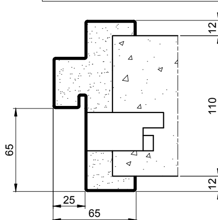
HUISSERIE ISOPHONIQUE \geq 110
