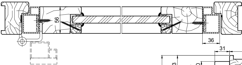
COUPE B-B SUR JOINT ANTI PINCE DOIGTS
