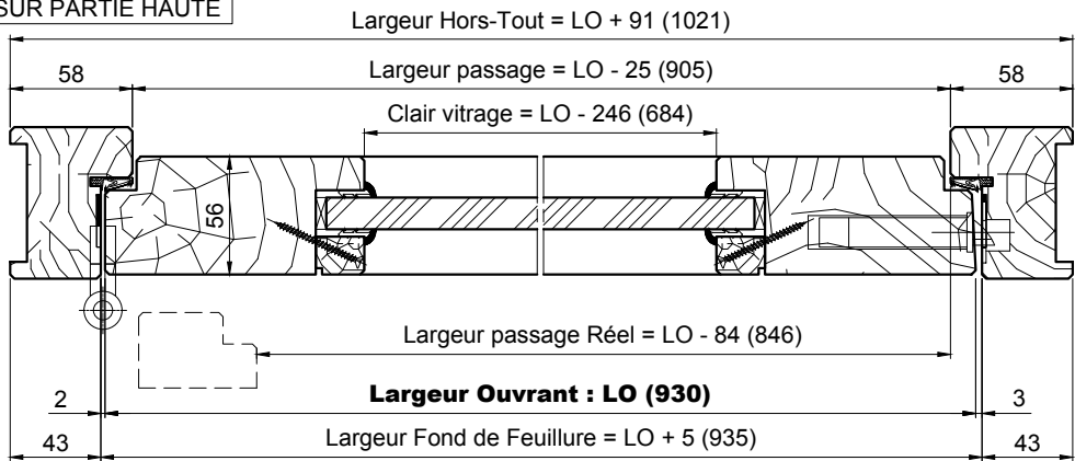
COUPE B-B SUR JOINT ANTI PINCE DOIGTS
