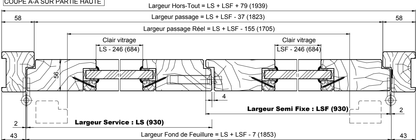
COUPE B-B SUR JOINT ANTI PINCE DOIGTS
