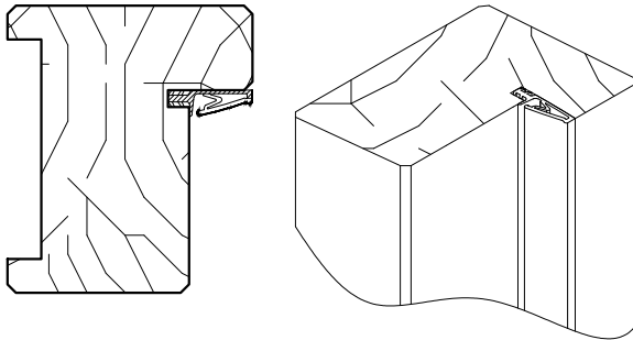
Profil avec joint ISO
