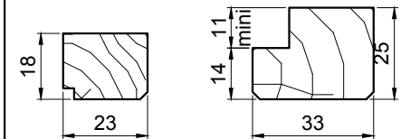
Sections des parclosos
