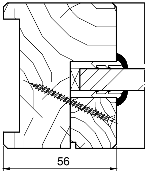
Simple parclosage
