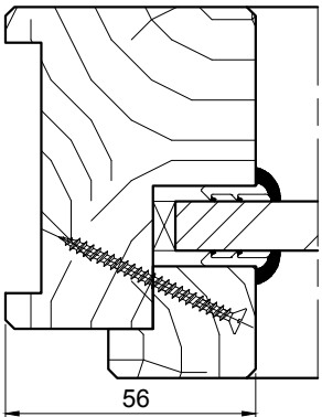
Simple parclosage
