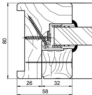
Parclosage avec fixation invisible
