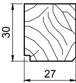
Sections des parcloes
