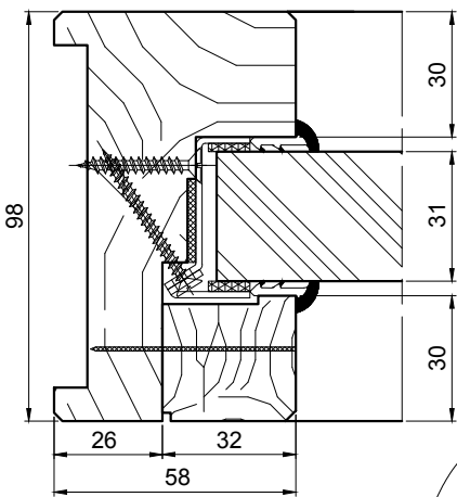
Parclosage avec fixation invisible
