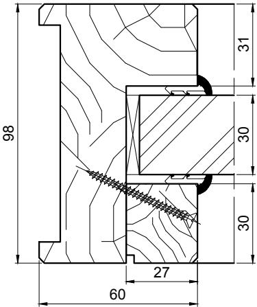
Simple parclosage
