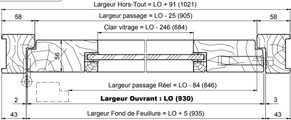
COUPE B-B SUR JOINT ANTI PINCE DOIGTS
