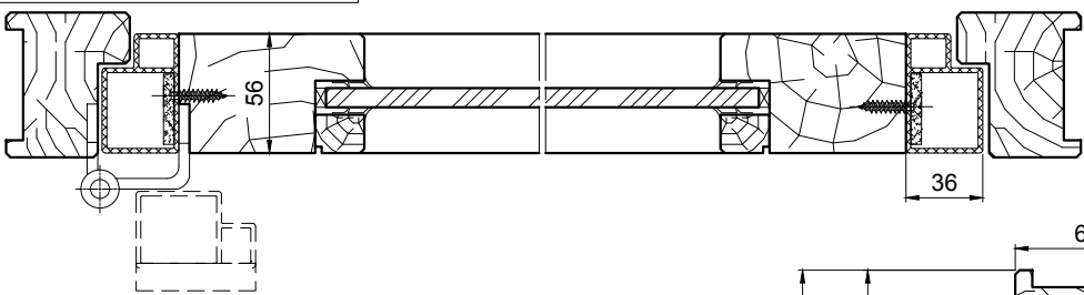
COUPE B-B SUR JOINT ANTI PINCE DOIGTS
