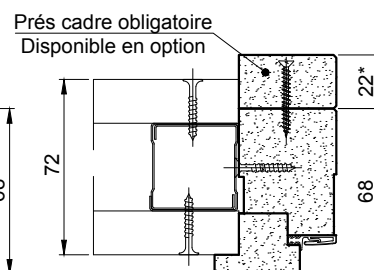
Schéma n°2 Pose à l'avancement
