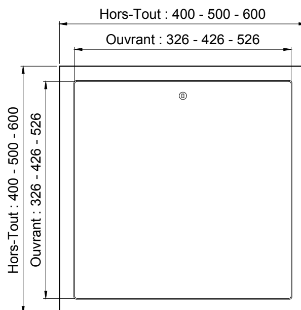
Schéma n°1 Pose après coup
