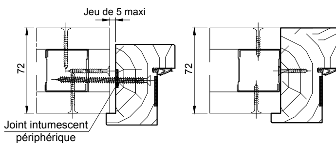
Schéma n°2 Pose à l'avancement
