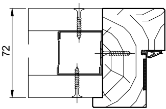
Schéma n°2 Pose à l'avancement
