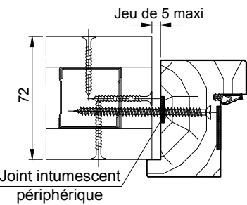
Schéma n°1 Pose après coup
