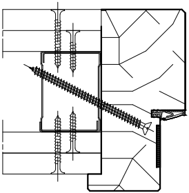
Schéma n°2 Pose à l'avancement
