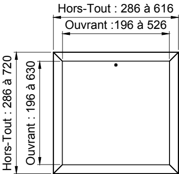
Schéma n°1 Pose après coup
