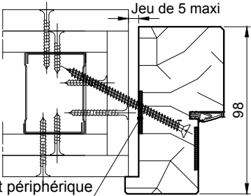
Schéma n°1 Pose après coup
