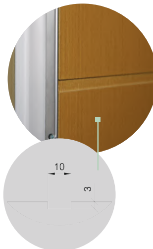
Coupe d'une rainure SYLVER Pour plus d'information, voir fiche technique MMO-028 et MMO-029
